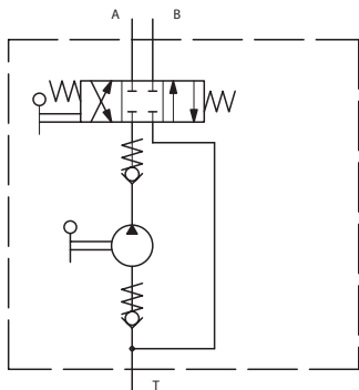
doppelwirkende Version (dw) ohne DBV
