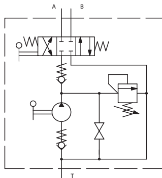
doppelwirkende Version (dw) mit DBV
